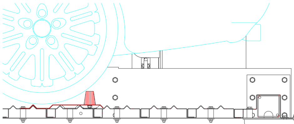
Rysunek 2 Auto parkujące tyłem z zamontowanym ogranicznikiem.
