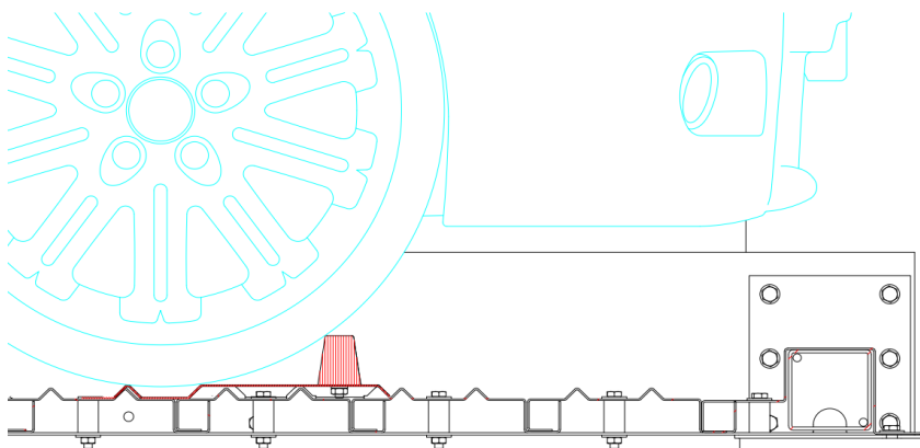
Rysunek 1 Auto parkujące przodem z zamontowanym ogranicznikiem.
