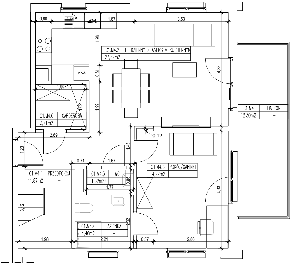
Poziom 1
